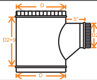
5. INJERTO ZAPATO REDONDO
