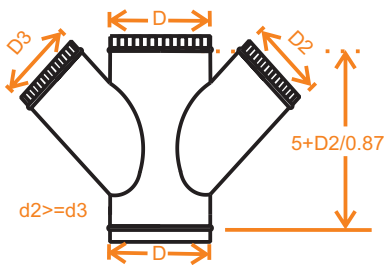
10. CRUZ REDONDA 45°
