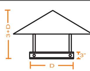
15. GORRO CHINO
