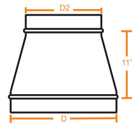
30. REDUCCIÓN CONCÉNTRICA
