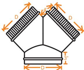
28. YEE
