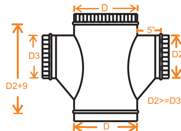
11. CRUZ ZAPATO REDONDO
