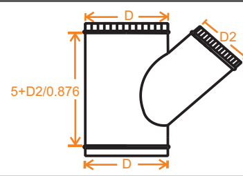
6. INJERTO 45°
