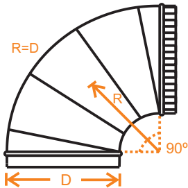
25. CODO 90
