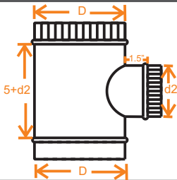
4. INJERTO REDONDO
