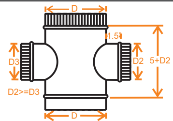
9. CRUZ REDONDA 90°
