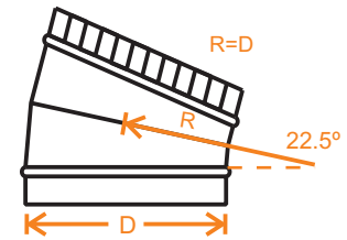
21. CODO 22.5
