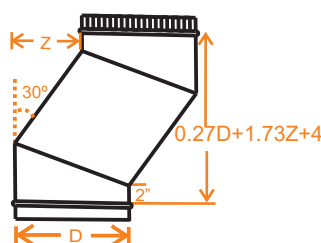
29. DESVIACIÓN
