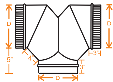
27. TEE ORIGINAL
