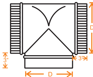
26. TEE ECONÓMICA
