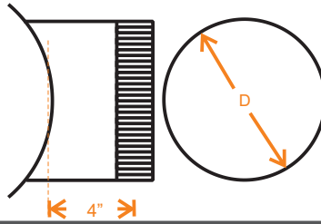
17. CASQUILLO REDONDO
