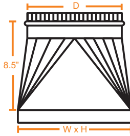
2. TRANSFORMACIÓN
