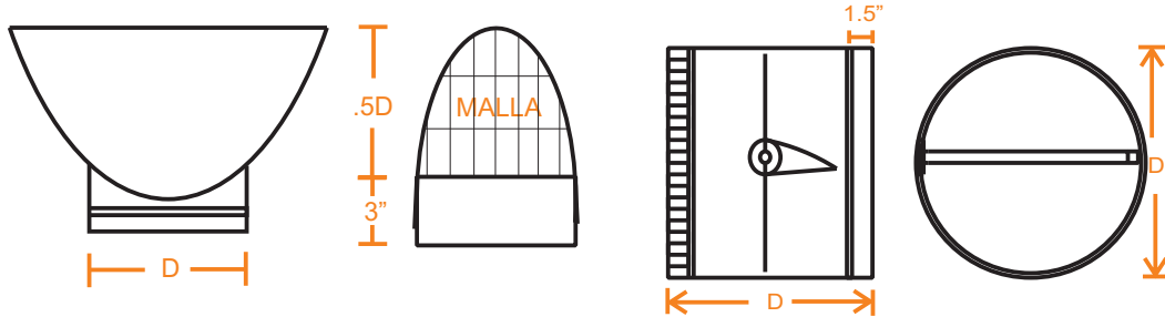
31. GORRO TACO
