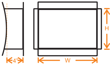
16. CASQUILLO CUADRADO
