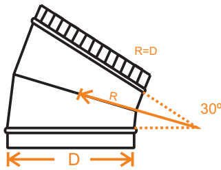
22. CODO 30
