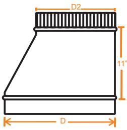
1. REDUCCIÓN EXCÉNTRICA
